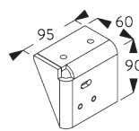
SG 8608 Plafondpoelie linkersteun
