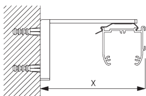
Smart Fix SG 11200 - SG 11205 en steun SG 2616: Schroef SG 10395 (M4x6) nodig.
