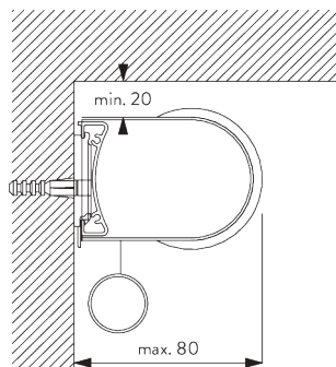
Bevestigingsprofiel SG 10534 en clicksteun SG 10539 Niet mogelijk met twee gekoppelde systemen!
