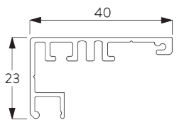
SG 11418 Zijgeleidingsprofiel
