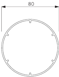
SG 11003 Profiel
