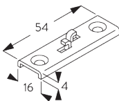
SG 6124 Steun
